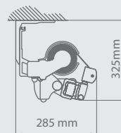
Mennyezeti beépítés
