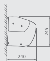
Falra szerelés
