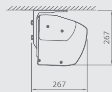
Mennyezeti beépítés
