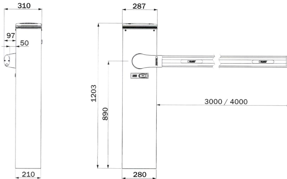
Sorompó méretei [mm]
